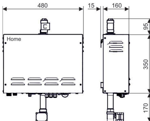
Abb. 4 Tylö Dampferzeuger Typ Home, Maßangaben in Millimetern
