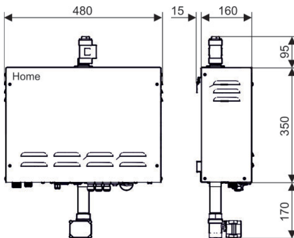
Rys. 4 Wytwnica pary Tył do użytku domowego; wymiary w milimetrach
