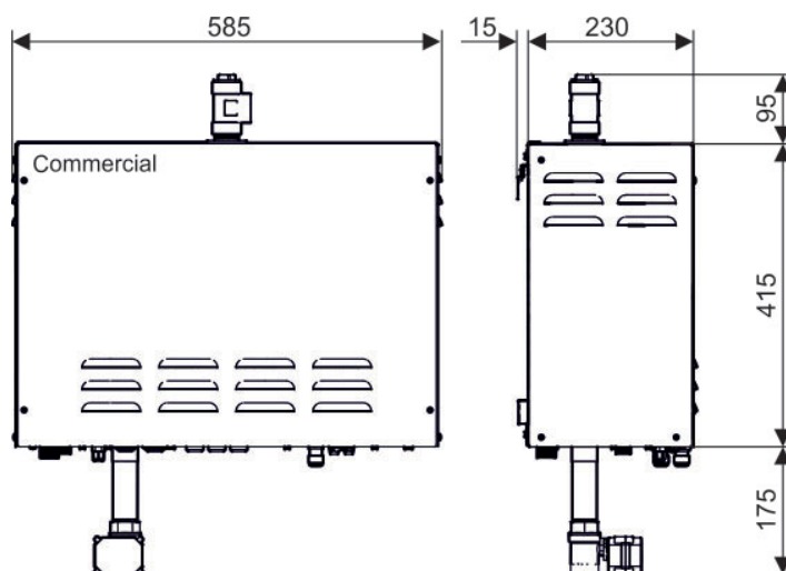
Abb. 5 Tylö Dampferzeuger Typ Commercial, Maßangaben in Millimetern
