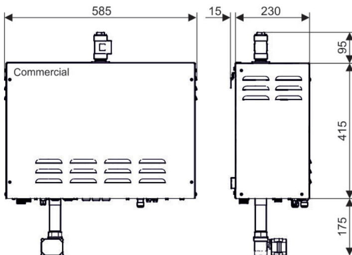
Rys. 5 Wytwnica pary Tył do użytku komercyjnego; wymiary w milimetrach
